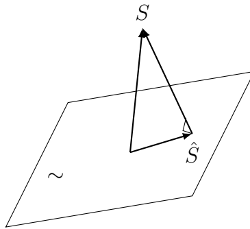
Figure 1.1: Interpretazione geometrica dell'ortogonalità: l'errore di stima è ortogonale al piano delle osservazioni.
